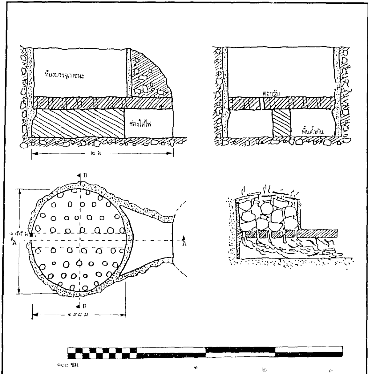
ภาพเส้นของเตาหมายเลข ๖๐ เป็นเตาชนิดระบายความร้อนผ่านในแนวดิ่งหรือเตาตะแกรง ซึ่งชุดเข้าไปในเนินดินของเตาหมายเลข ๓๔ จากแหล่งเตาบ้านเกาะน้อย อำเภอศรีสัชนาลัย จังหวัดสุโขทัย
