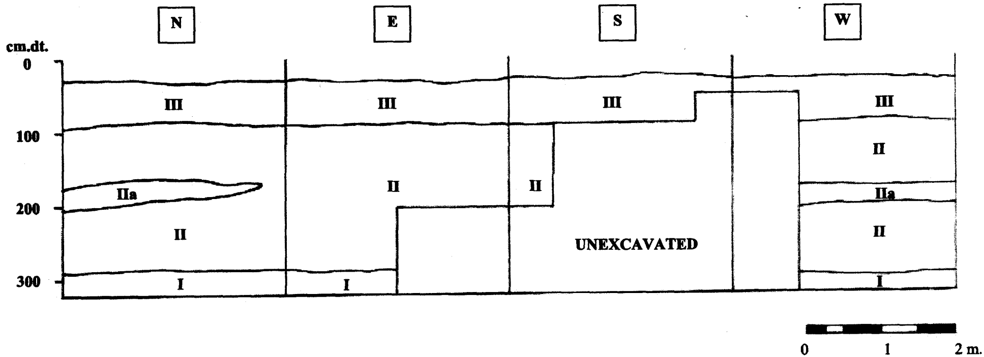
แผนผังที่ ๑ ผังชั้นดิน PIT 1
