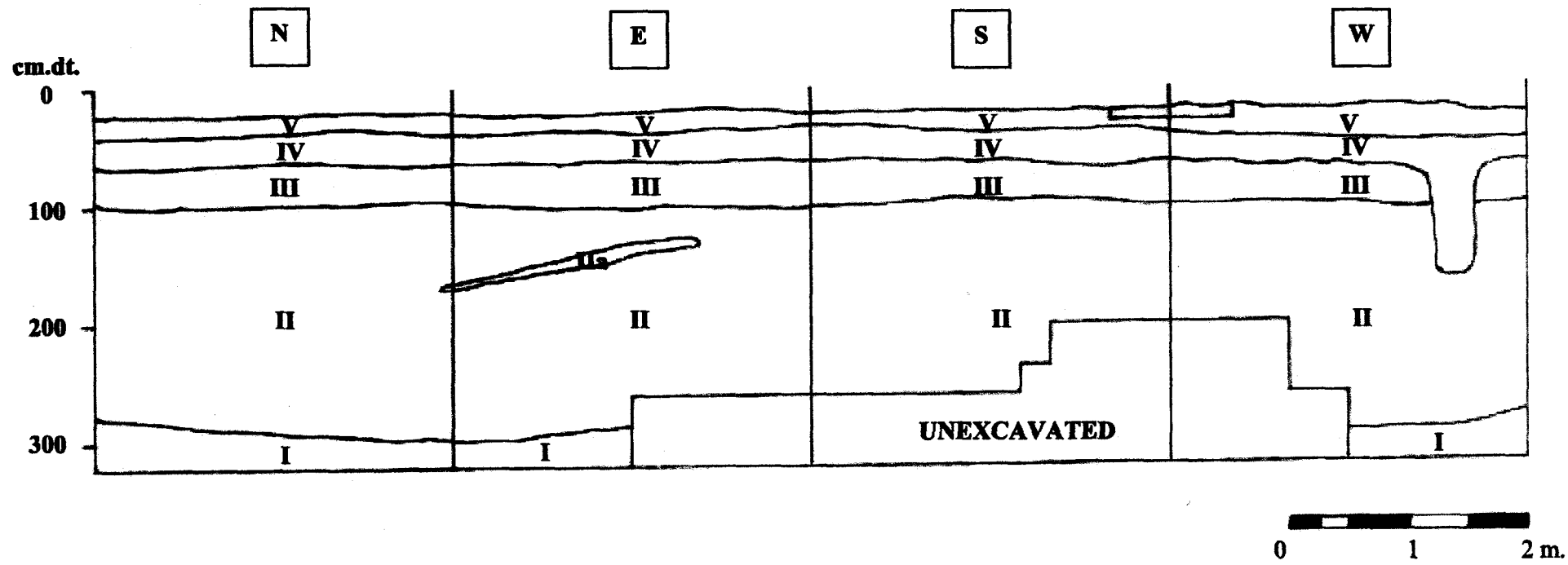
แผนผังที่ ๒ ผังชั้นดิน PIT 2
