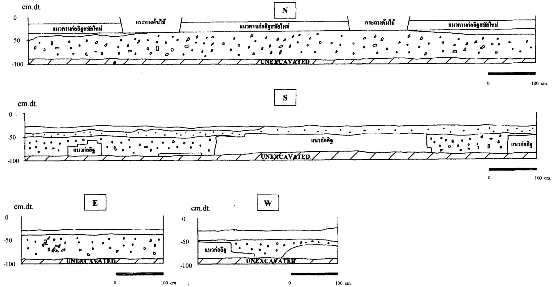
ภาพลายเส้นที่ ๒๒ แสดงผังชั้นดิน หลุมขุดตรวจหาแนวโบราณสถานหมายเลข 14
