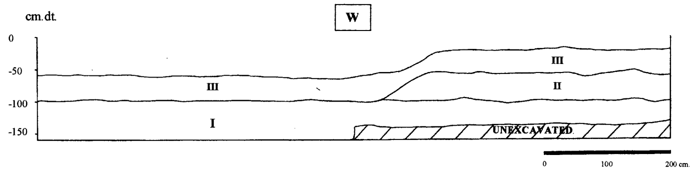
ภาพลายเส้นที่ ๕ แสดงผังชั้นดิน หลุมขุดตรวจหาแนวโบราณสถานหมายเลข 1 ด้านทิศตะวันออกและตะวันตก
