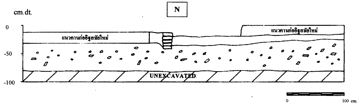
ภาพลายเส้นที่ ๒๑ แสดงผังชั้นดิน หลุมขุดตรวจหาแนวโบราณสถานหมายเลข 13
