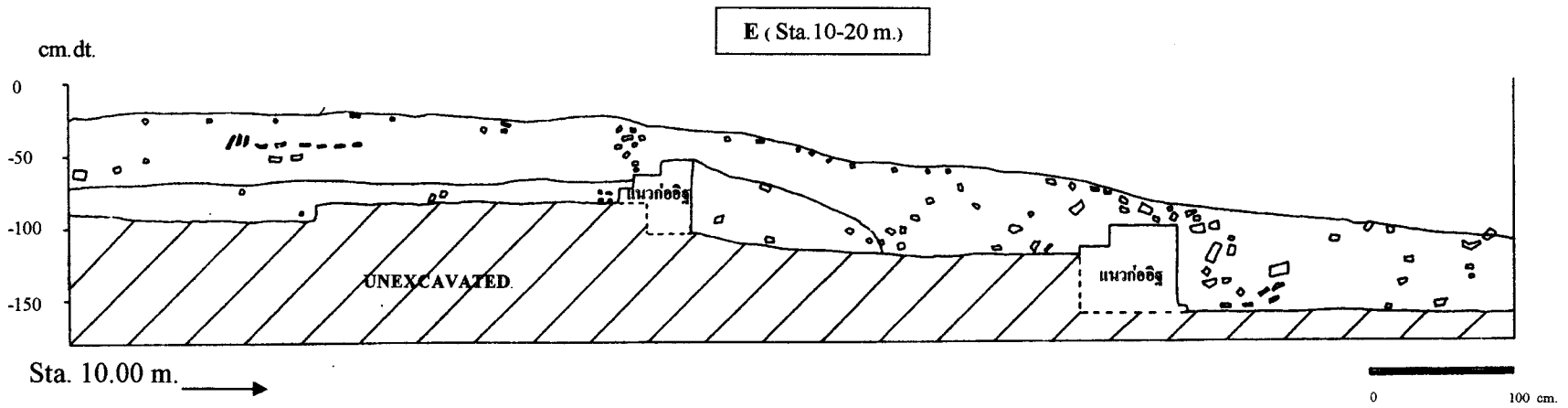
ภาพถ่ายเส้นที่ ๑๒ แสดงผังชั้นดิน หลุมขุดตรวจหาแนวโบราณสถานหมายเลข 4 ด้านทิศตะวันออก
