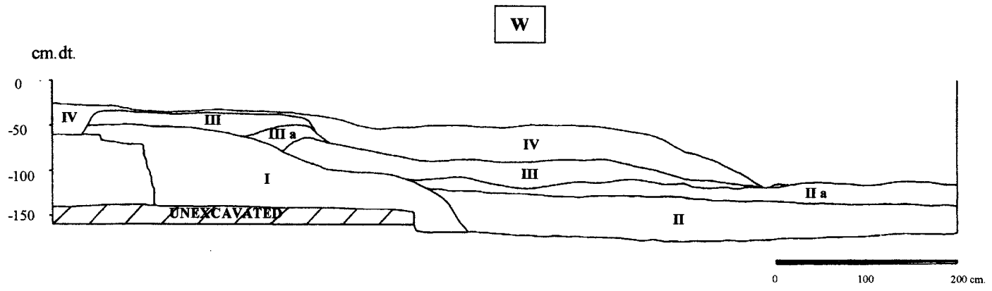
ภาพลายเส้นที่ ๗ แสดงผังชั้นดิน หลุมขุดตรวจหาแนวโบราณสถานหมายเลข 2 ด้านทิศตะวันออกและตะวันตก
