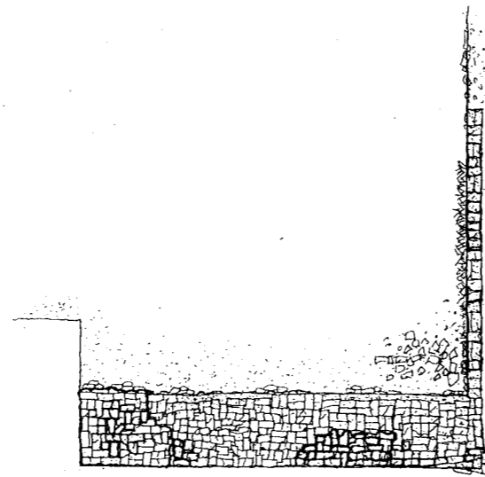
รูปแปลน หลุมขุดตรวจแนวโบราณสถาน หมายเลข ๖
