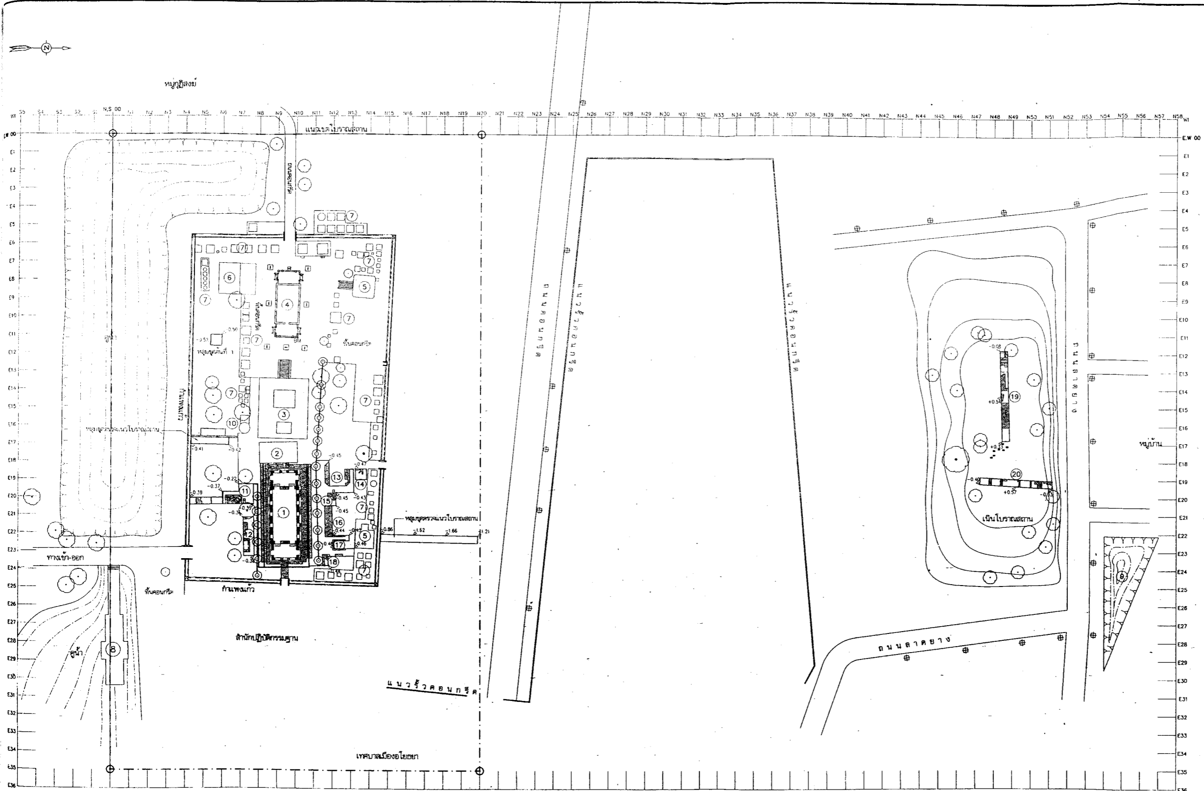
ผังแสดงตำแหน่งพื้นที่หลังการขุดแต่งและหลุมขุดตรวจแนวโบราณสถาน มณฑลอุดร 1:500
