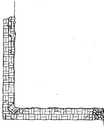
รูปแปลน หลุมขุดตรวจแนวโบราณสถาน หมายเลข ๘ มาตราส่วน 1:50
