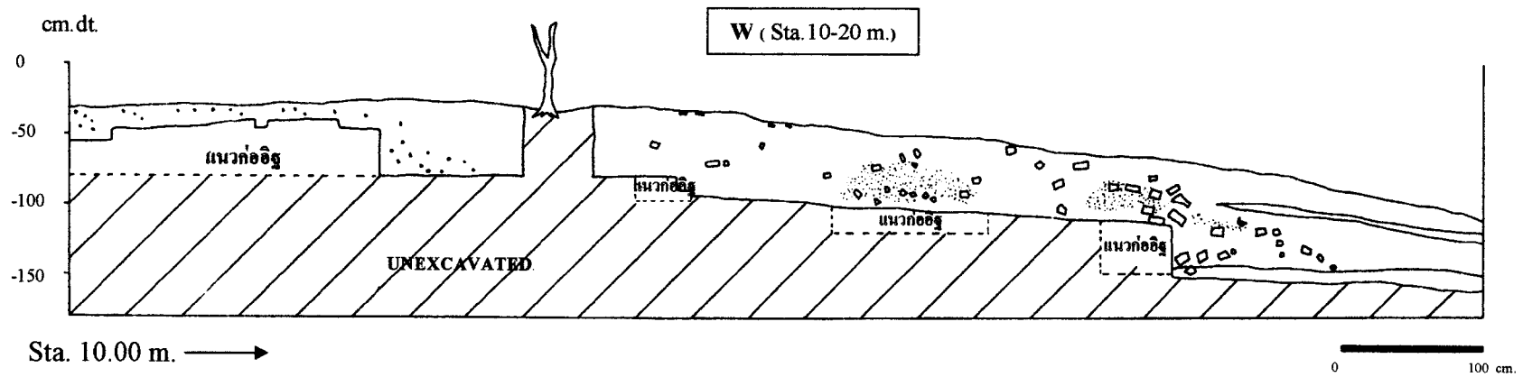
ภาพลายเส้นที่ ๑๓ แสดงผังชั้นดิน หลุมขุดตรวจหาแนวโบราณสถานหมายเลข 4 ด้านทิศตะวันตก
