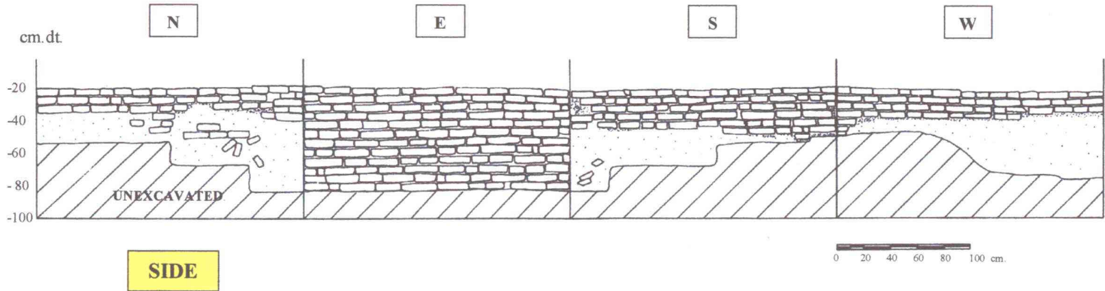
ภาพถ่ายต้นที่ ๑ แสดงผังชั้นดิน หลุมขุดตรวจที่ 1
