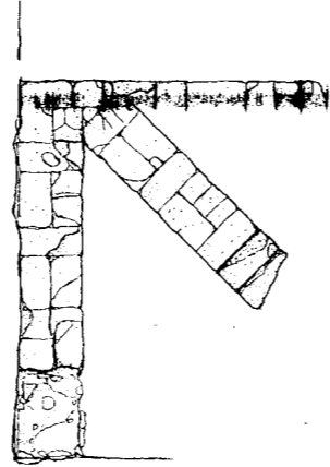
รูปแปลน หลุมขุดตรวจแนวโบราณสถาน หมายเลข ๔ มาตราส่วน 1 : 20
