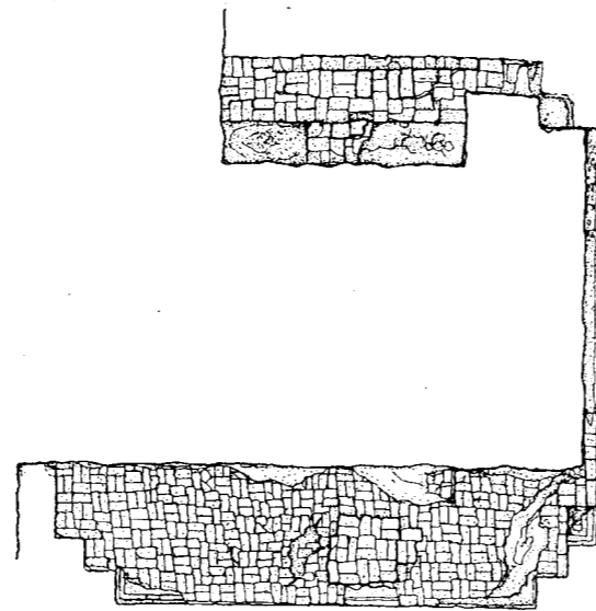
รูปแปลน หลุมขุดตรวจแนวโบราณสถาน หมายเลข ๓ มาตราส่วน 1:50
