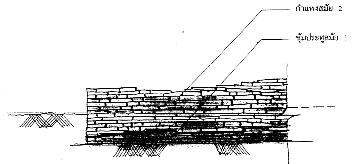
แบบขยาย A 4
