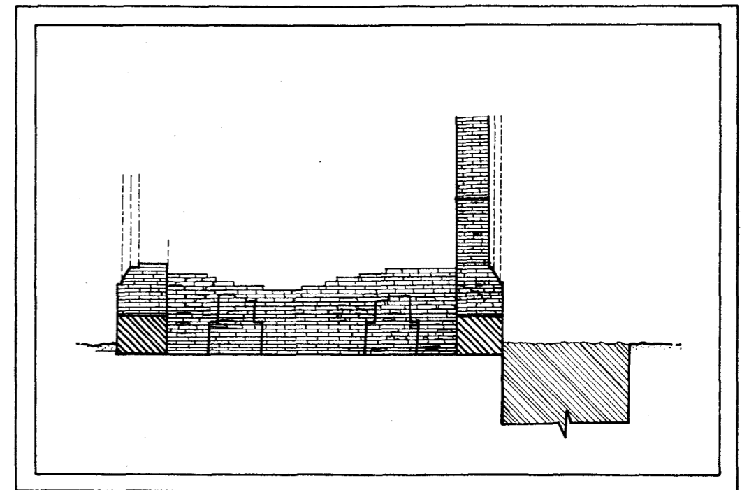
ภาพตัดแสดงการยึดดินเพื่อก่อสร้างอาคารตำหนัก บริเวณหลุมขุดค้น T.P.1 ด้านทิศใต้ติดผนังภายนอก
