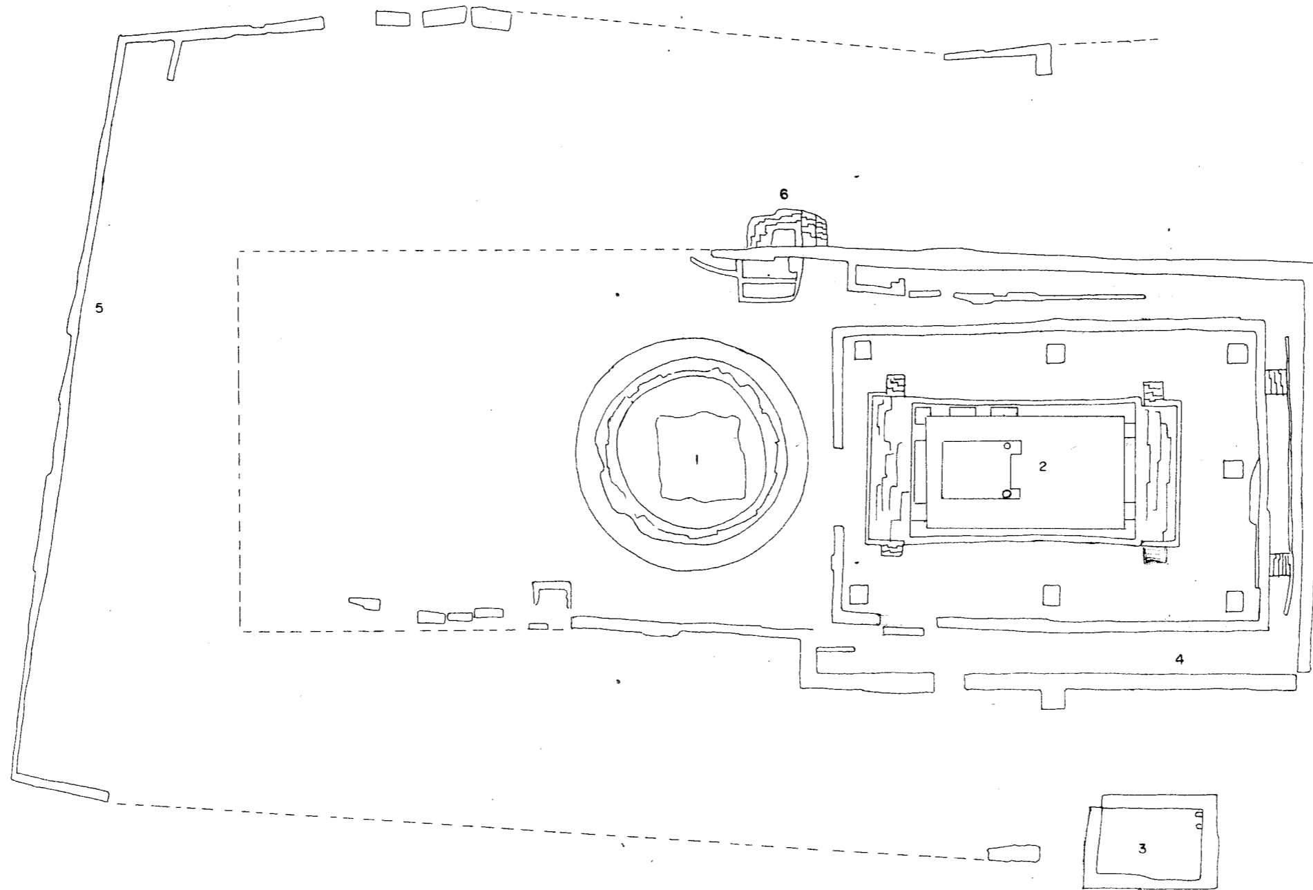
แผนผังที่ 1. ผังบริเวณวัดสมัยที่ 2 (วัดสีกาตมุต) สภาพหลังการขุดแต่ง
