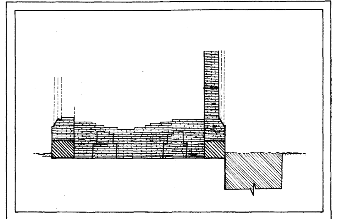
ภาพตัดแฉกแสดงการยึดดินเพื่อก่อสร้างอาคารตำหนัก บริเวณหลุมขุดค้น T.P.1 ด้านทิศใต้ติดผนังภายนอก
