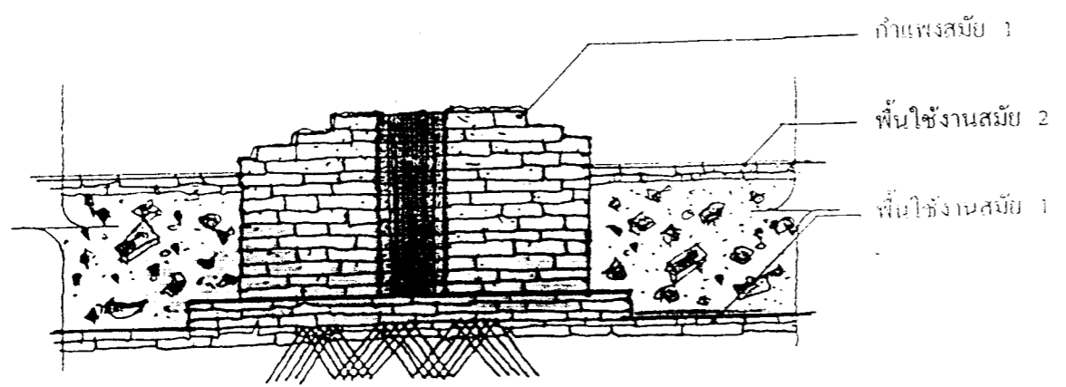
แบบขยาย A 1
