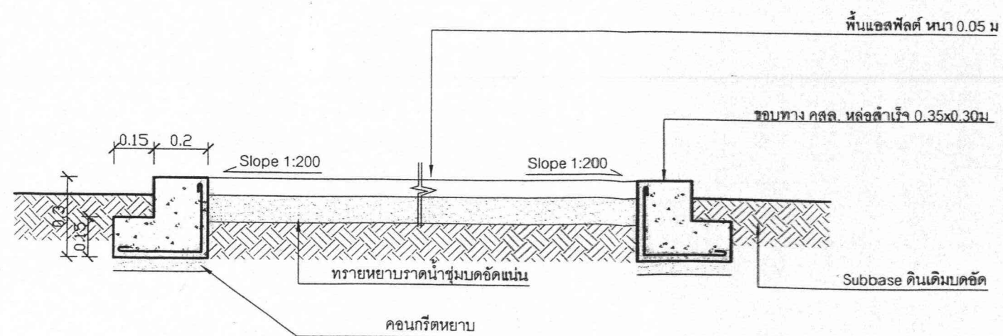
รูปตัดตามขวาง มาตราส่วน 1:20
