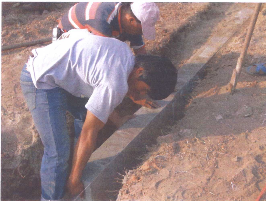
ขณะดำเนินการขุดวางคาน ค.ส.ล.สำเร็จรูป
