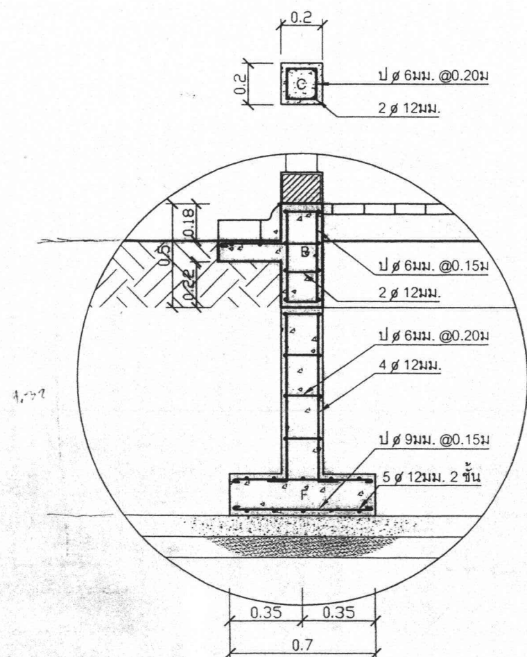
แบบขยายโครงสร้างใต้ดิน มาตราส่วน 1:25
