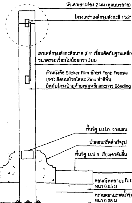
รูปตัดตามขวาง มาตราส่วน 1:10
