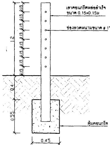
รูปตัด มาตราส่วน 1:25
