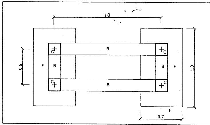
แปลนโครงสร้างใต้ดิน มาตราส่วน 1:25
