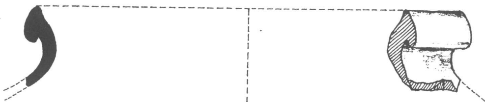
ภาพลายเส้นที่ 19 ปากกระปุก เตาแม่น้ำน้อย พบในระดับ 280-290Cm.Dt.
