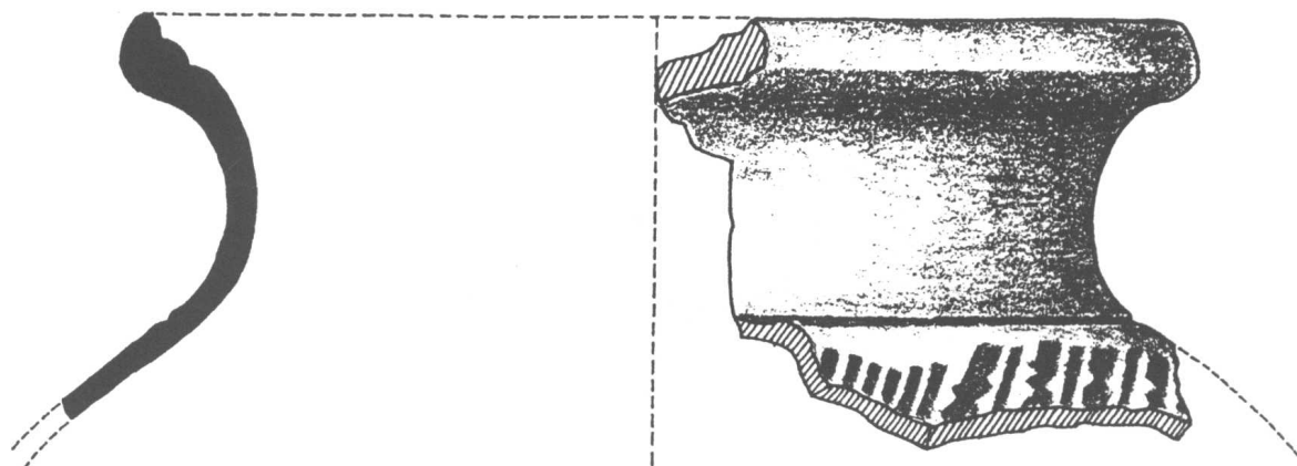
ภาพลายเส้นที่ 29 ปากหม้อทะนนวนโค้งออก ลาย 6 เนื้อดินธรรมดา พบในระดับ 200-210 Cm.Dl.
