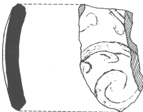
ภาพลายเส้นที่ 9 ตัวตลับ ขูดลายพันธุ์พฤกษาใต้เคลือบ เตาศรีสังขาลย์ พบในระดับ 160-170 Cm.Dt.
