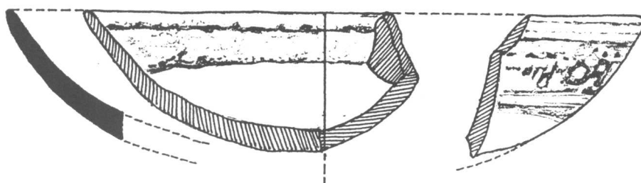
ภาพลายเส้นที่ 17 ปากขามเคลือบเขียวใส เตาศรีสังขนาลัย พบในระดับ 290-300 Cm.Dt.
