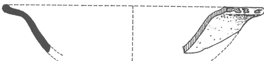
ภาพลายเส้นที่ 24 ปากขามเขียนลายดำได้เคลือบ เตาถ่านนา พบในระดับ 330-340 Cm.Dt.
