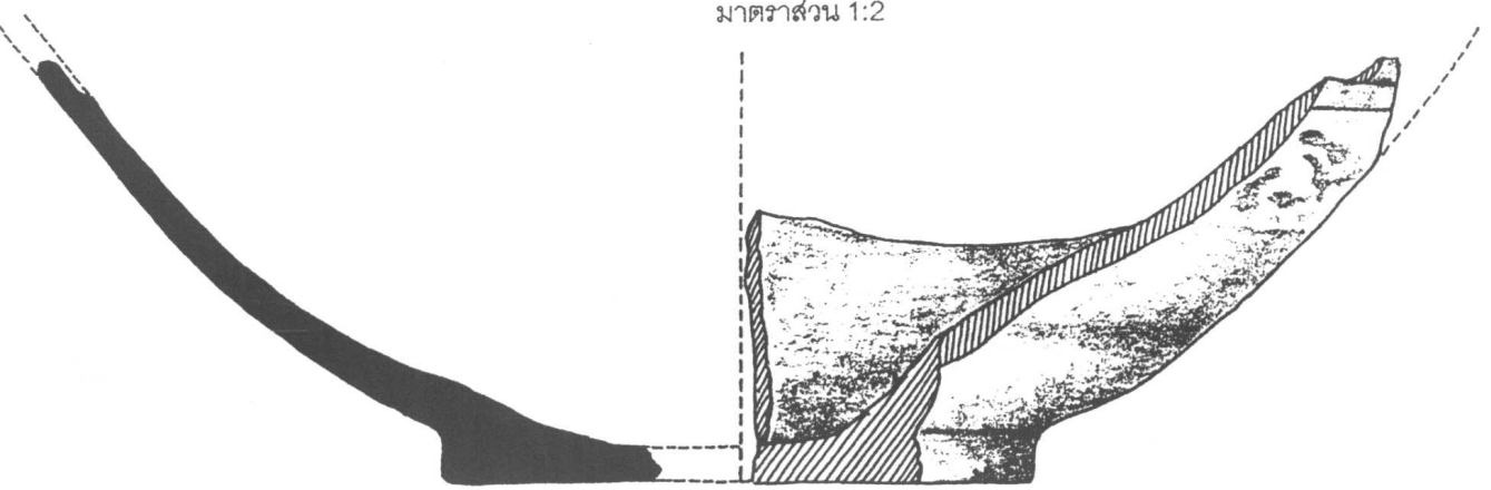
ภาพลายเส้นที่ 33 ก้นขาม เนื้อดินธรรมดา พบในระดับ 300-310 Cm.Dl.
