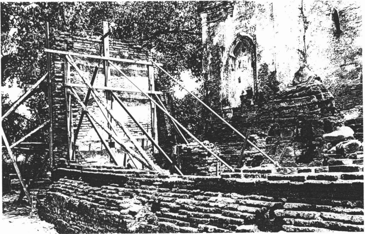
รูปที่ 103 เสริมความมั่นคงผนังมุขปราสาททิศตะวันตกด้านในเพิ่มเติม
