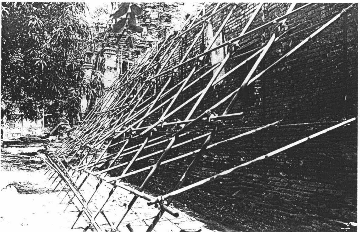
รูปที่ 102 เสริมความมั่นคงผนังวิหารด้านทิศตะวันตกด้วยโครงเหล็ก
