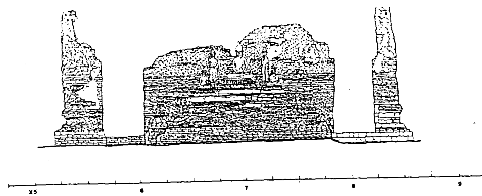
รูปตั้งทิศตะวันตก วัดพระมหาธาตุ (5)
