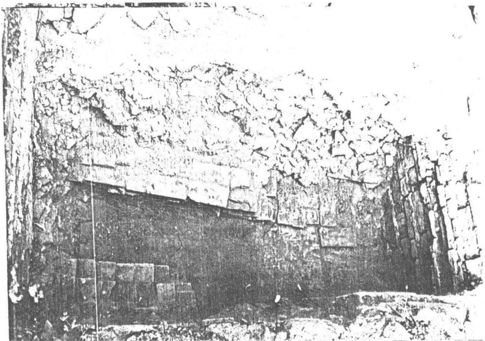
ภาพที่ 10 ลักษณะของรากฐานปรารักษ์ใช้อิฐก่อเป็นรากฐานชั้นล่าง
