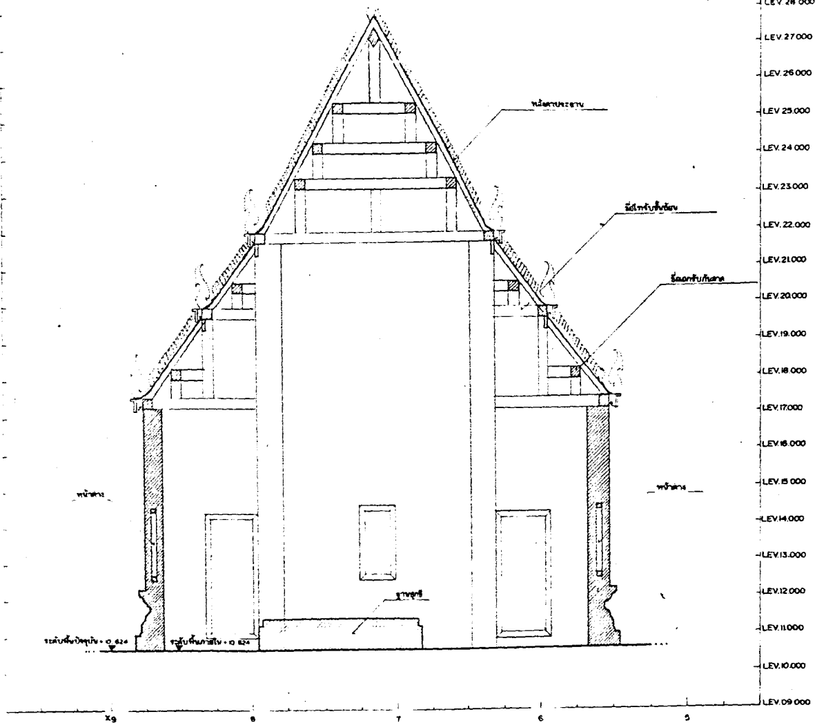
รูปตัดตามขวาง วิหารทนายเลข(๕)(รูปสันนิษฐาน)
