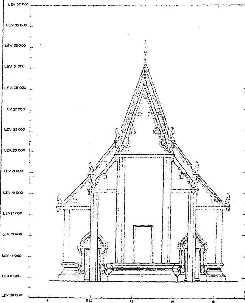
รูปตั้ง กิเลสวันออก อุโบสถ หมายเลข② รูปสันนิษฐาน
