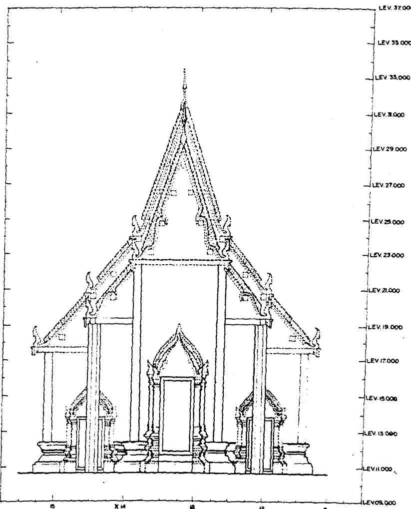
รูปตั้ง กิเลสวันตก อุโบสถ หมายเลข② รูปสันนิษฐาน
