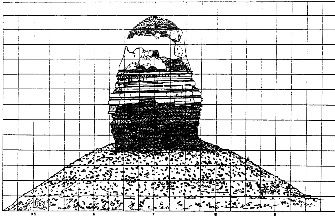
รูปตั้งทิศตะวันออก, เจดีย์ทรงระฆังคว่ำ พนมมณ ๔
