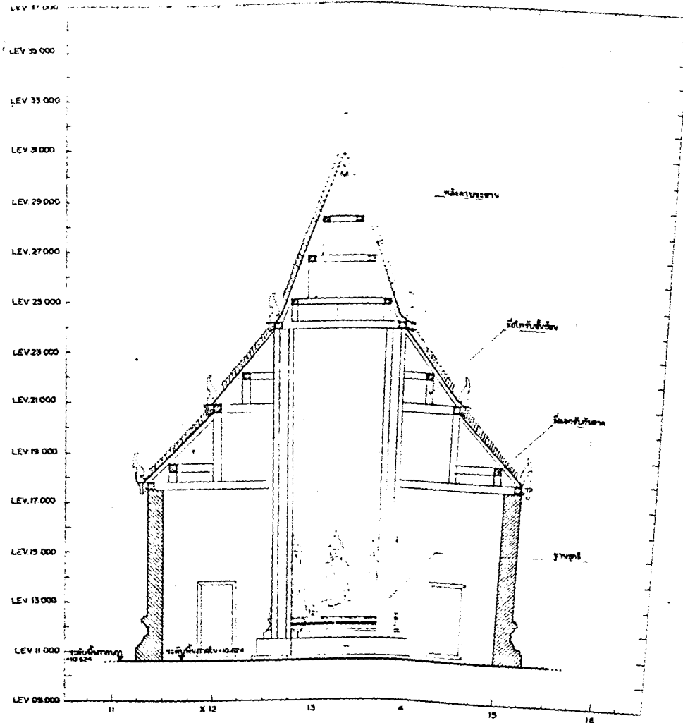
รูปตัดตามขวาง อุโบสถ (วัดบ้านไร่)
