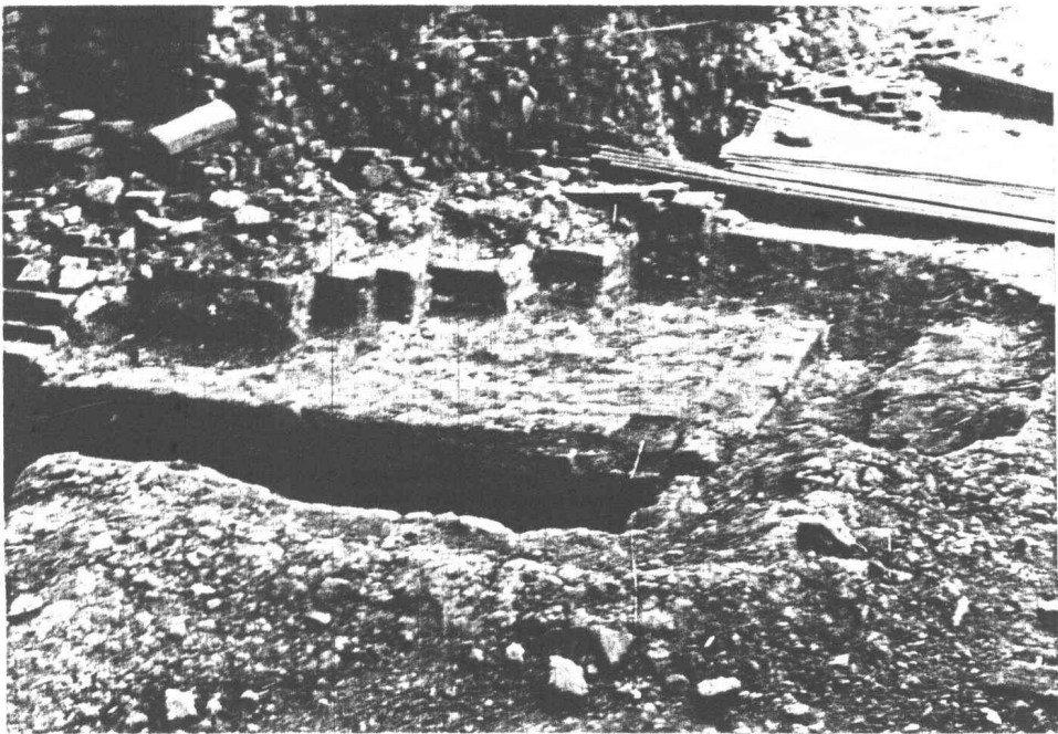
ภาพที่ 27 ลักษณะการก่ออิฐเป็นรากฐานสี่เหลี่ยมก่อนที่จะถึงฐานย่อมุม เจดีย์ทรงปราสาท
