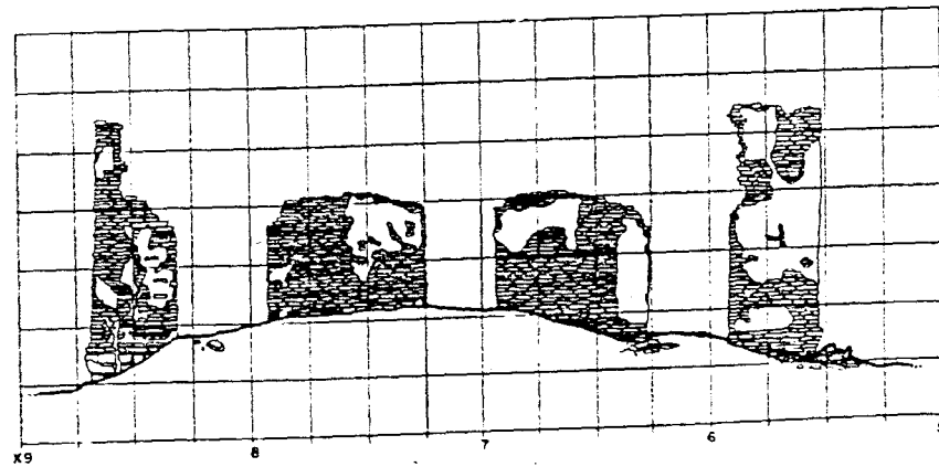
รูปตั้งทิศตะวันตก วัดพระแก้วมรกต ๕
