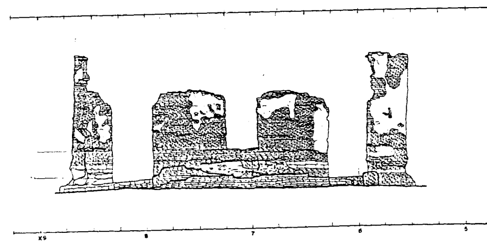
รูปตั้งทิศตะวันตก วัดพระมหาธาตุ (5)
