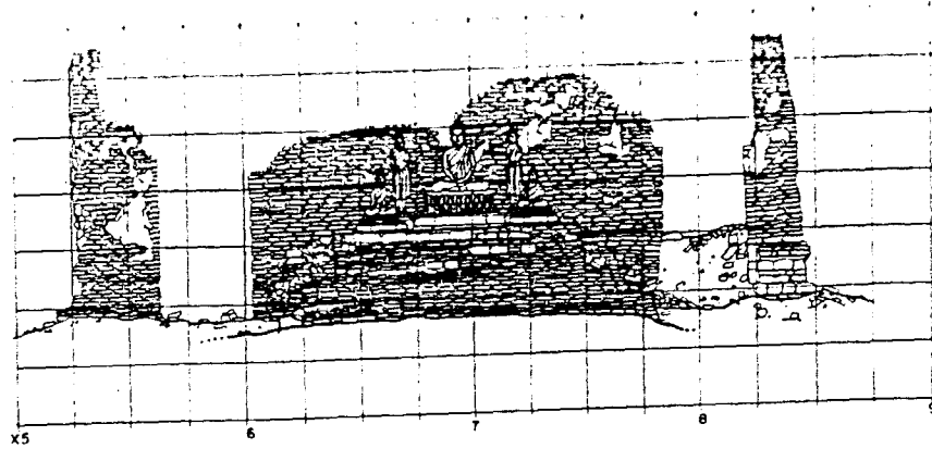
รูปตั้งทิศตะวันตก วัดพระแก้วมรกต ๕
