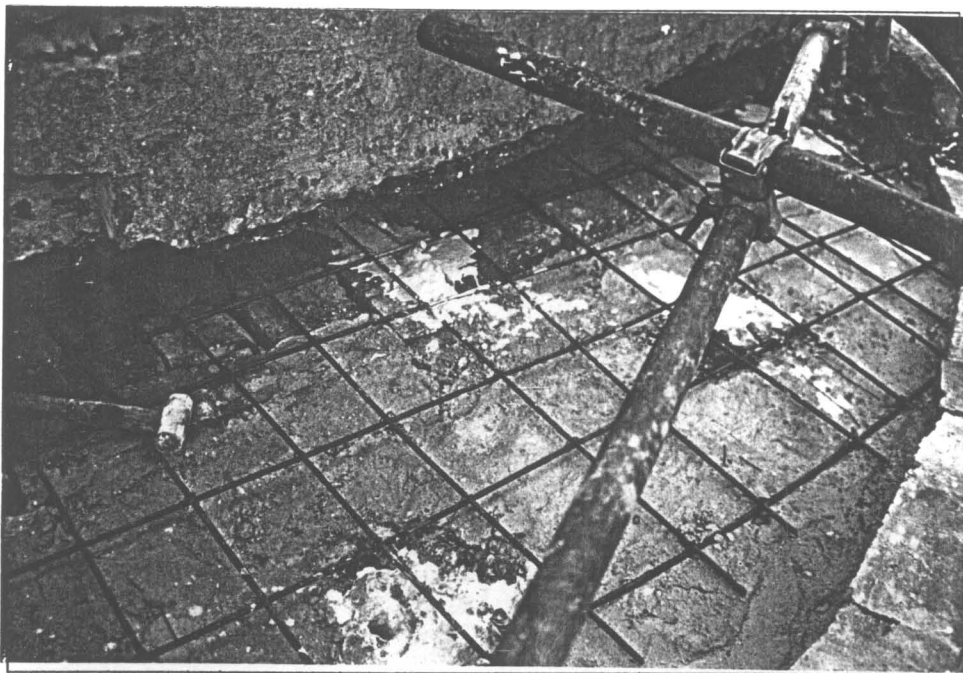
รูปที่ 79 วางตะแกรงเหล็ก เทคาน ค.ส.ล.ด้านบนของครุฑมั่ง (5/8)
