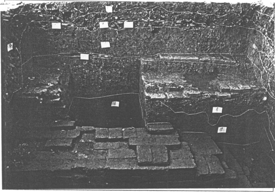
รูปที่ 61 ผังชั้นดินหลุมขุดค้น S2E13 (4/6)
