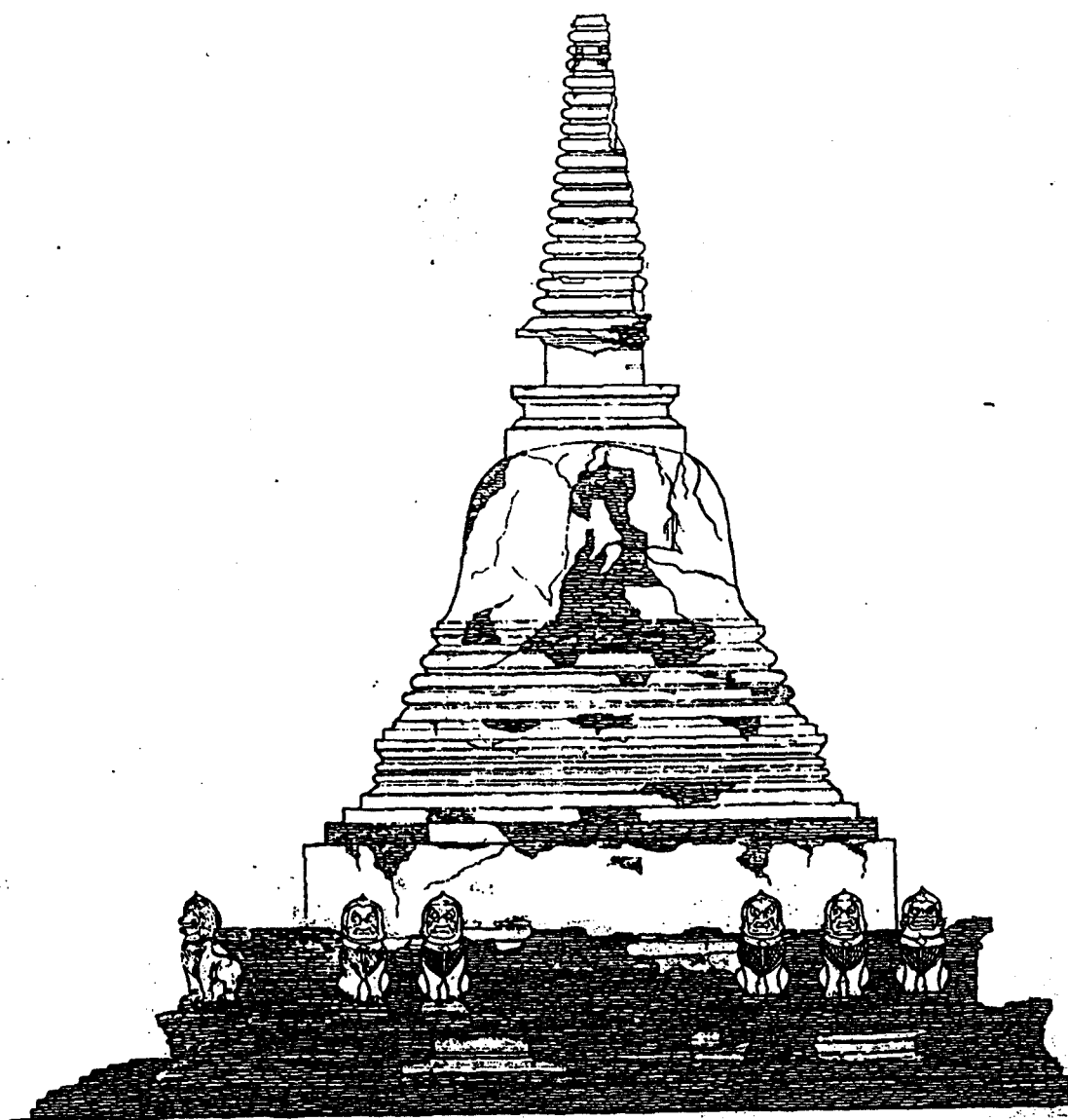
รูปด้าน เทวเทว มาตราส่วน 1 : 75
