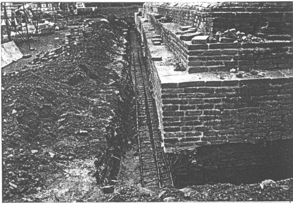
รูปที่ 74 วางเหล็ก เทคานค.ส.ล. รอบฐานเจดีย์ประธาน (3/11)
