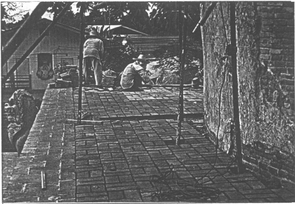
รูปที่ 78 ปูพื้นลานด้านบนทูดฐานบัวเหนือชั้นรองรับสิ่งปูผนัง (5/36)
