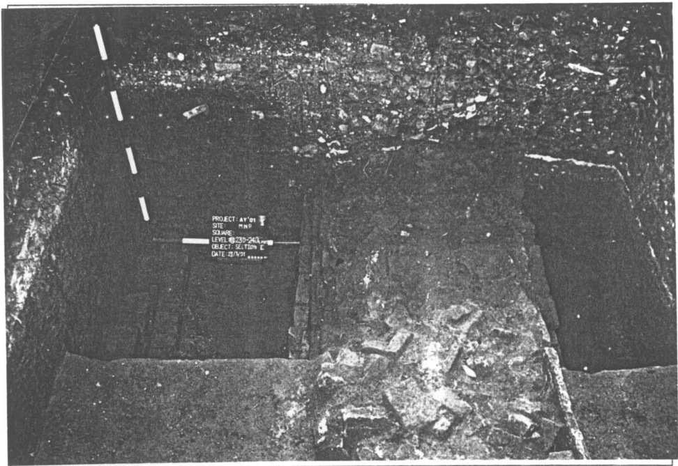
รูปที่ 12 สภาพหลุมขุดค้นระดับ ⑪ 230-240 (3/2)
