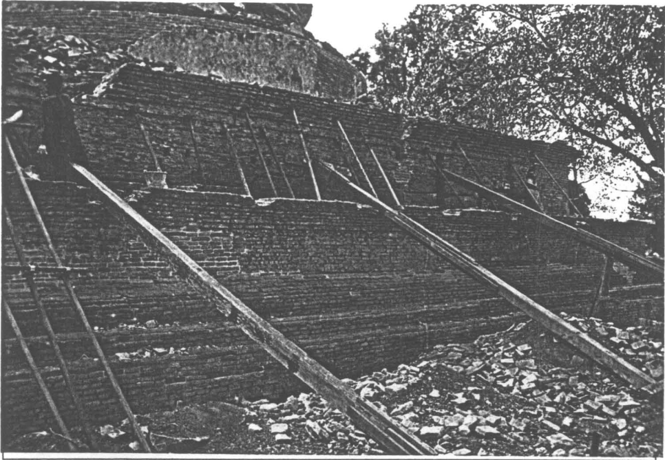
รูปที่ 75 ขณะผลัดต้นฐานบัวเหนือชั้นรองรับสิงห์ปูนปั้น (3/23)
