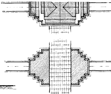
รูปแปลน ชุ่มประตู่ แบบวิเศษ มาตราส่วน 1 / 50
