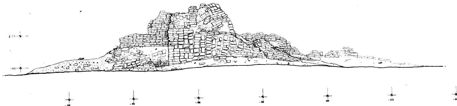
รูปด้าน วัดพระนาค มาตราส่วน 1 / 25
