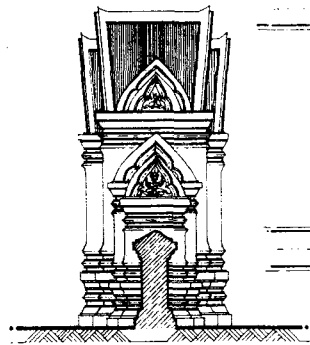
รูปด้านข้าง ชุ่มประตู่ แบบวิเศษ มาตราส่วน 1 / 50
