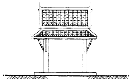
รูปด้านข้าง อาคารหมายเลข 6. แบบวิไลระห์. มาตราส่วน 1 / 50.
