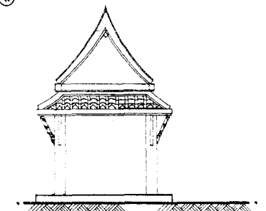
รูปด้านหน้า อาคารหมายเลข 6. แบบวิไลระห์. มาตราส่วน 1 / 50.
