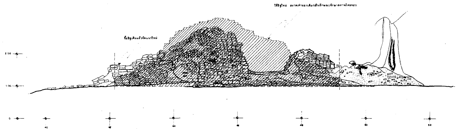
รูปด้าน ทิศใต้ มาตราส่วน 1 / 25
