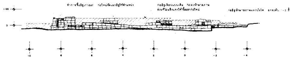
รูปด้าน ทิศตะวันตก มาตราส่วน 1 / 50
