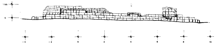
รูปด้าน ทิศตะวันตก มาตราส่วน 1 / 50
