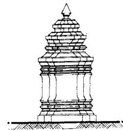
รูปด้าน เลาเม็ด แบบวิเศษ มาตราส่วน 1 / 50
