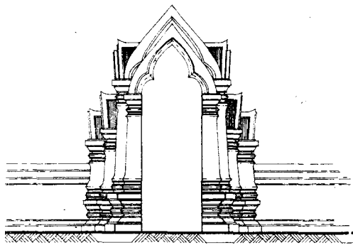
รูปด้านหน้า ชุ่มประตู่ แบบวิเศษ มาตราส่วน 1 / 50
