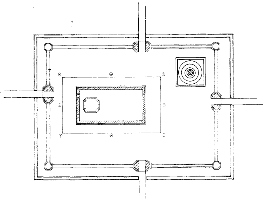
รูปผังบริเวณ โบสถ์, เจดีย์, ชุ่มประตู่, เลาเม็ด แบบวิเศษ มาตราส่วน 1 / 200
