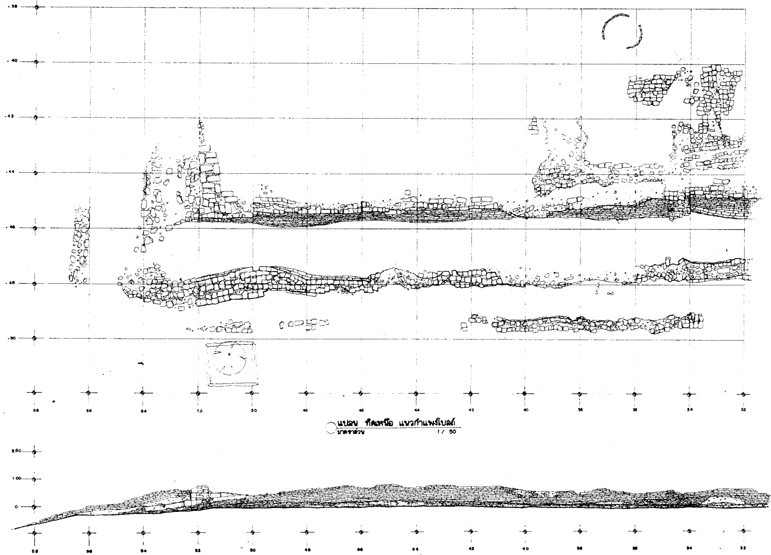
รูปด้าน ทิศเหนือ แนวกำแพงโบราณ มาตราส่วน 1/50
