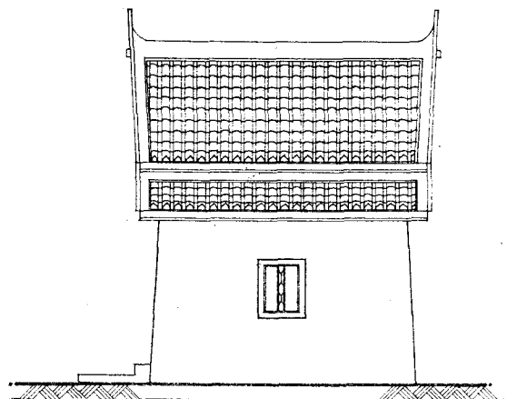
รูปด้านข้าง อาคารหมายเลข 5. แบบวิไลระห์. มาตราส่วน 1 / 50.
