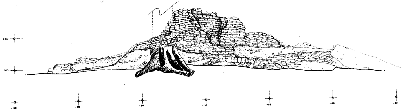
รูปด้าน วัดพระนอน มาตราส่วน 1 / 25
