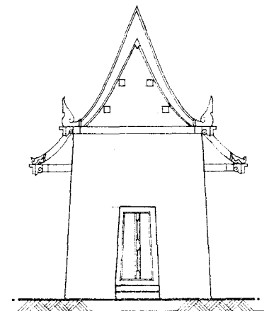
รูปด้านหน้า อาคารหมายเลข 5. แบบวิไลระห์. มาตราส่วน 1 / 50.
