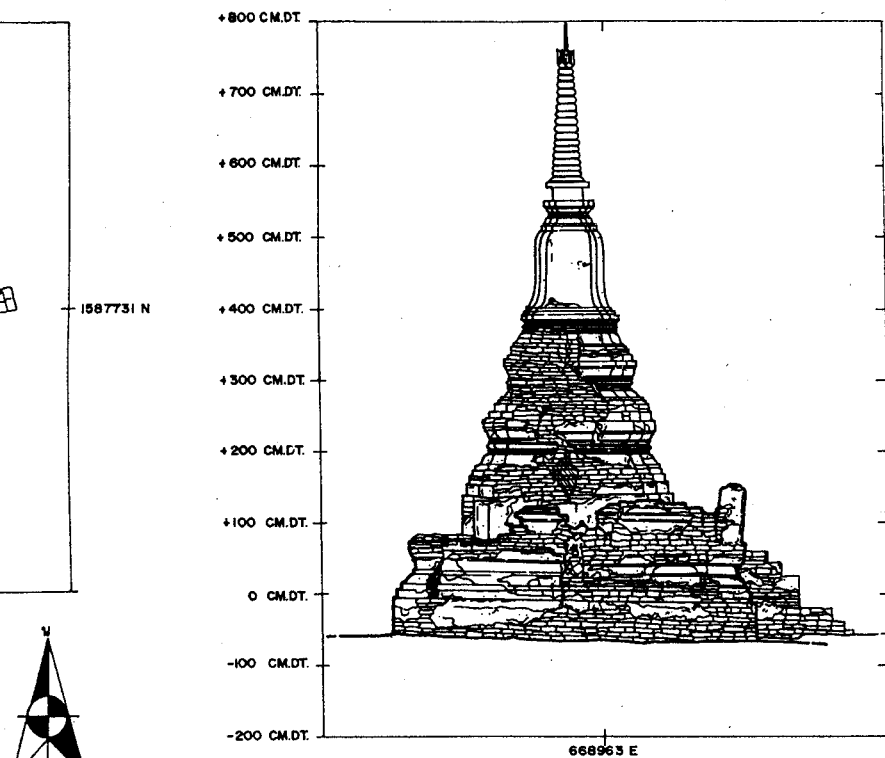
รูปด้านทิศใต้
