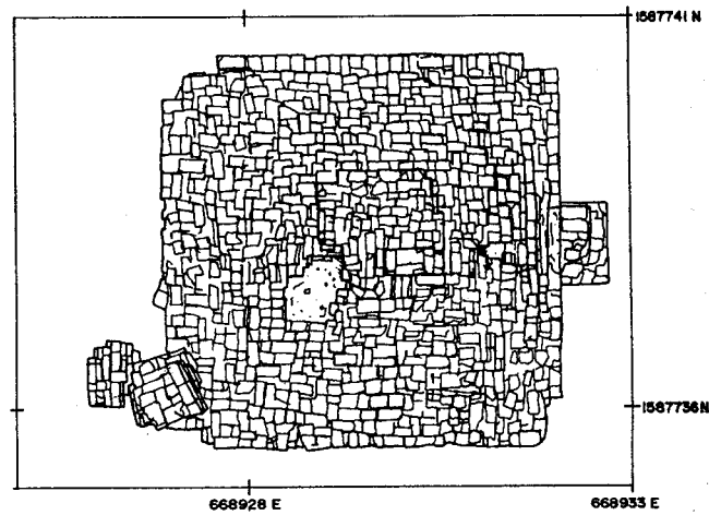
รูปผังพื้น เจดีย์ราย หมายเลข ๕
