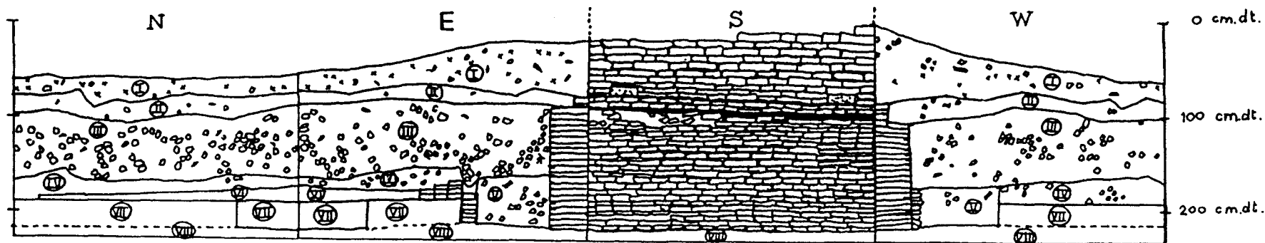
ผังชั้นดินหลุมขุดตรวจฐานเจดีย์ประธานด้านทิศเหนือ(กริดN3W1)
