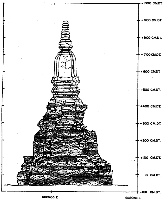
รูปด้านทิศเหนือ
